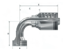
CAT Flange
