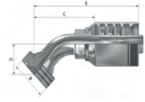
CAT Flange
