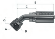
JIC F 37° Swivel
