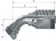
JIC F 37° Swivel
