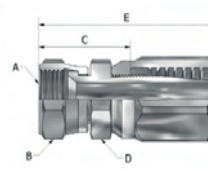
JIC F 37° Swivel
