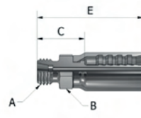
Metric M 24° Cone
