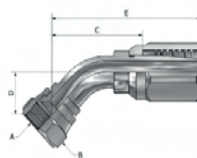
JIC F 37° Swivel
