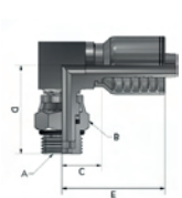
UNO Male Swivel
