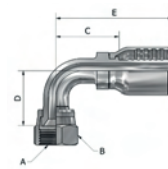
JIC F 37° Swivel
