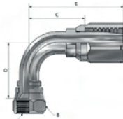
JIC F 37° Swivel
