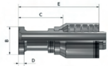
LeTourneau Flange
