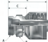
Metric M 24° Cone
