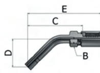
Stand Pipe
